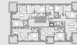
Plan général
