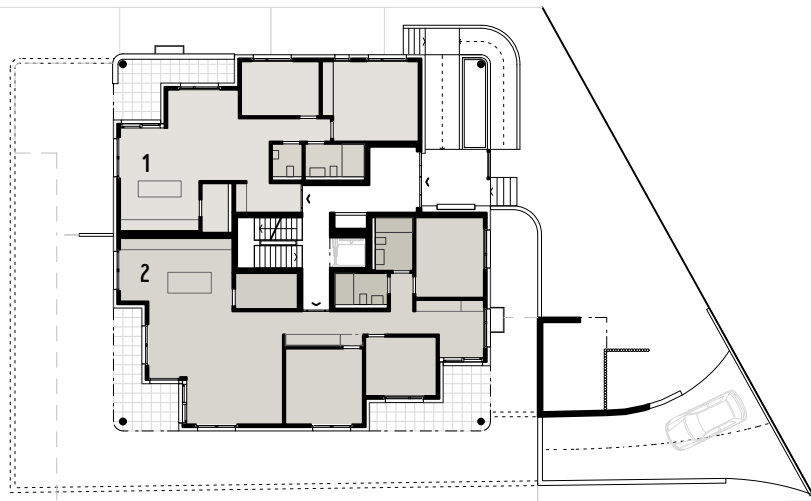
Erdgeschoss
