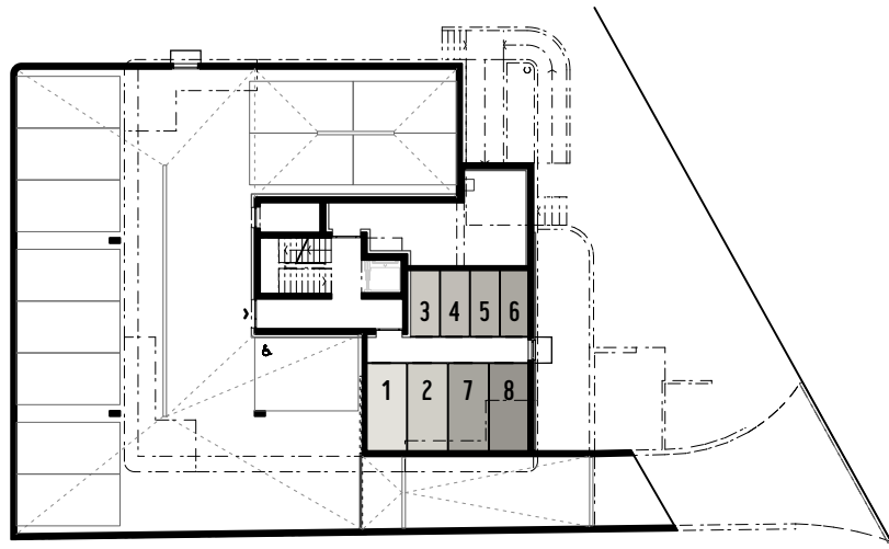
Untergeschoss
