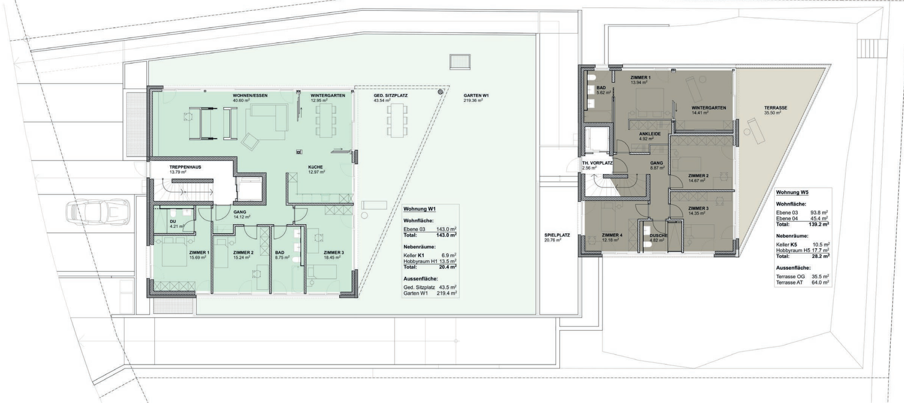
ERDGESCHOSS HAUS A
