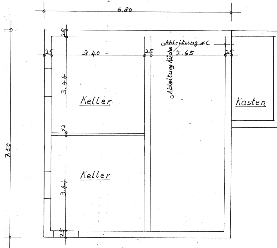
Grundriss Erdgeschoss
