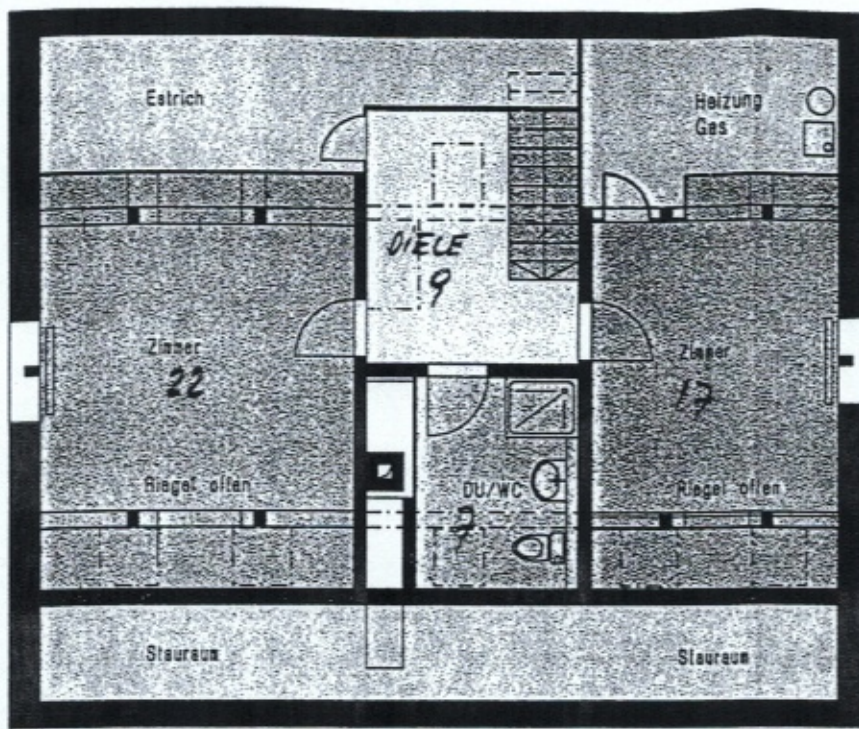
2. OBERGESCHOSS
