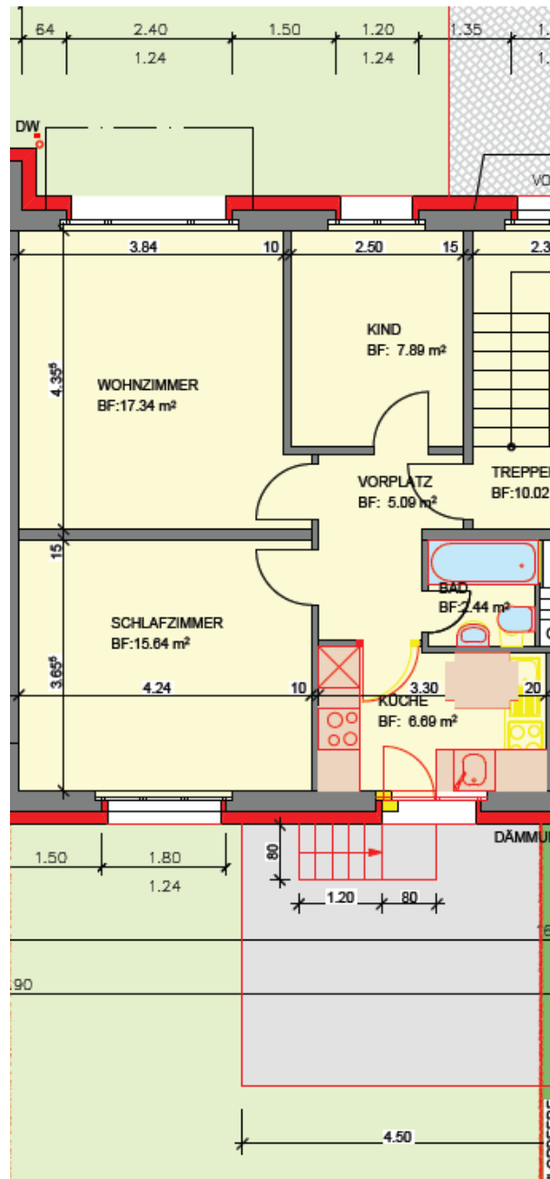
Mattenweg 2, 4415 Lausen 3-ZWG HP rechts mit Gartensitzplatz Mst 1:100
