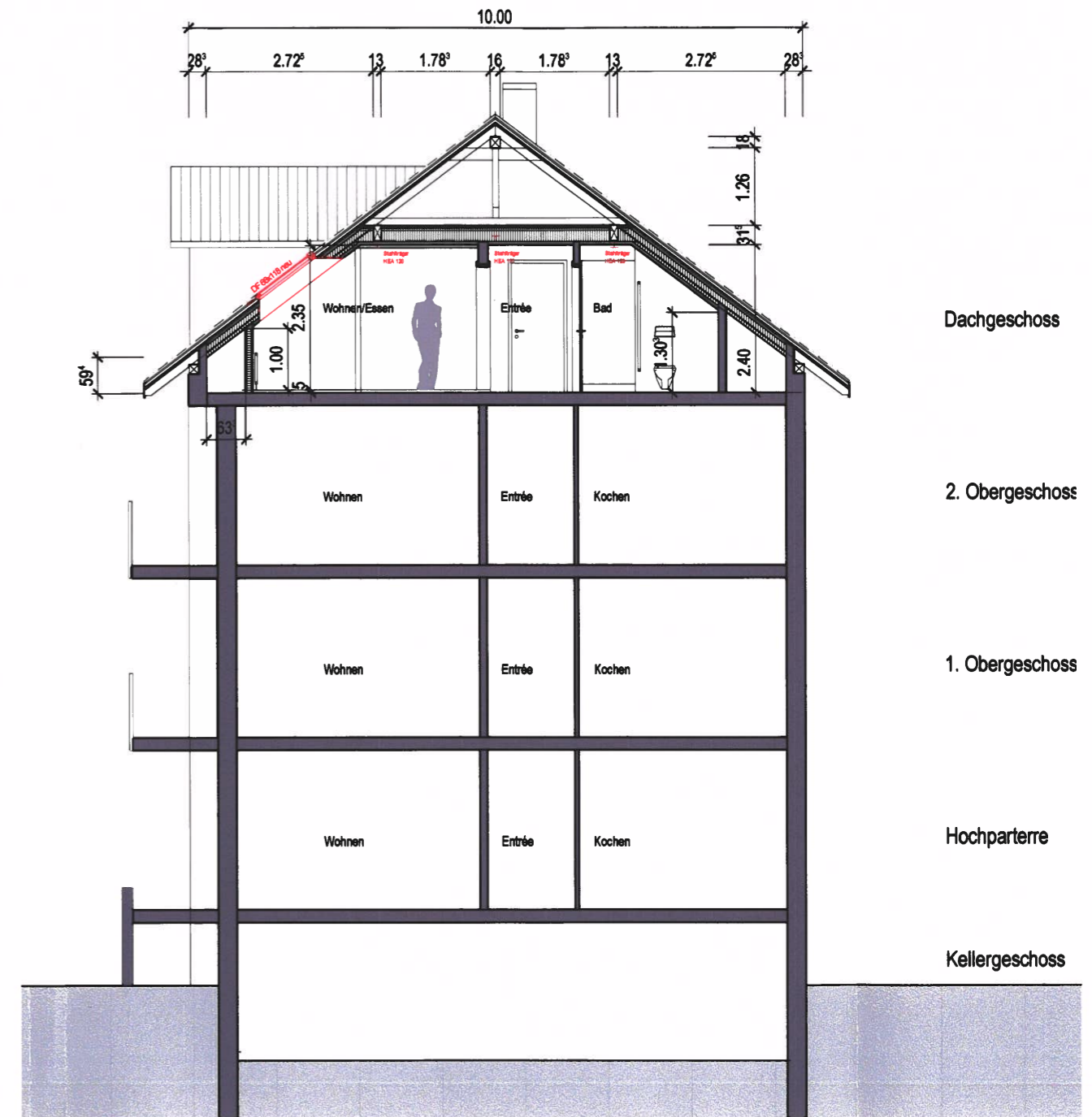
Schnitt A-A
