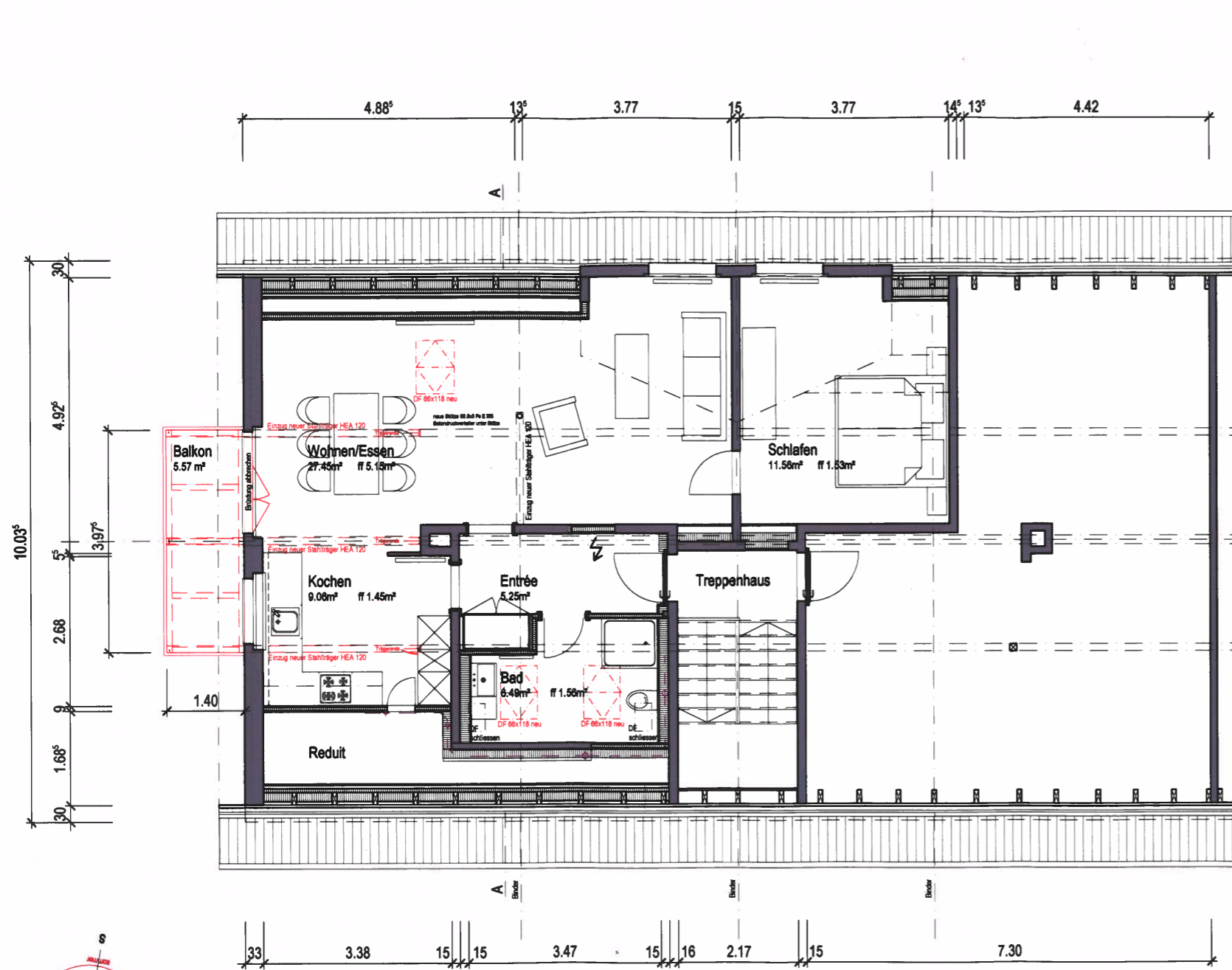
Grundriss
