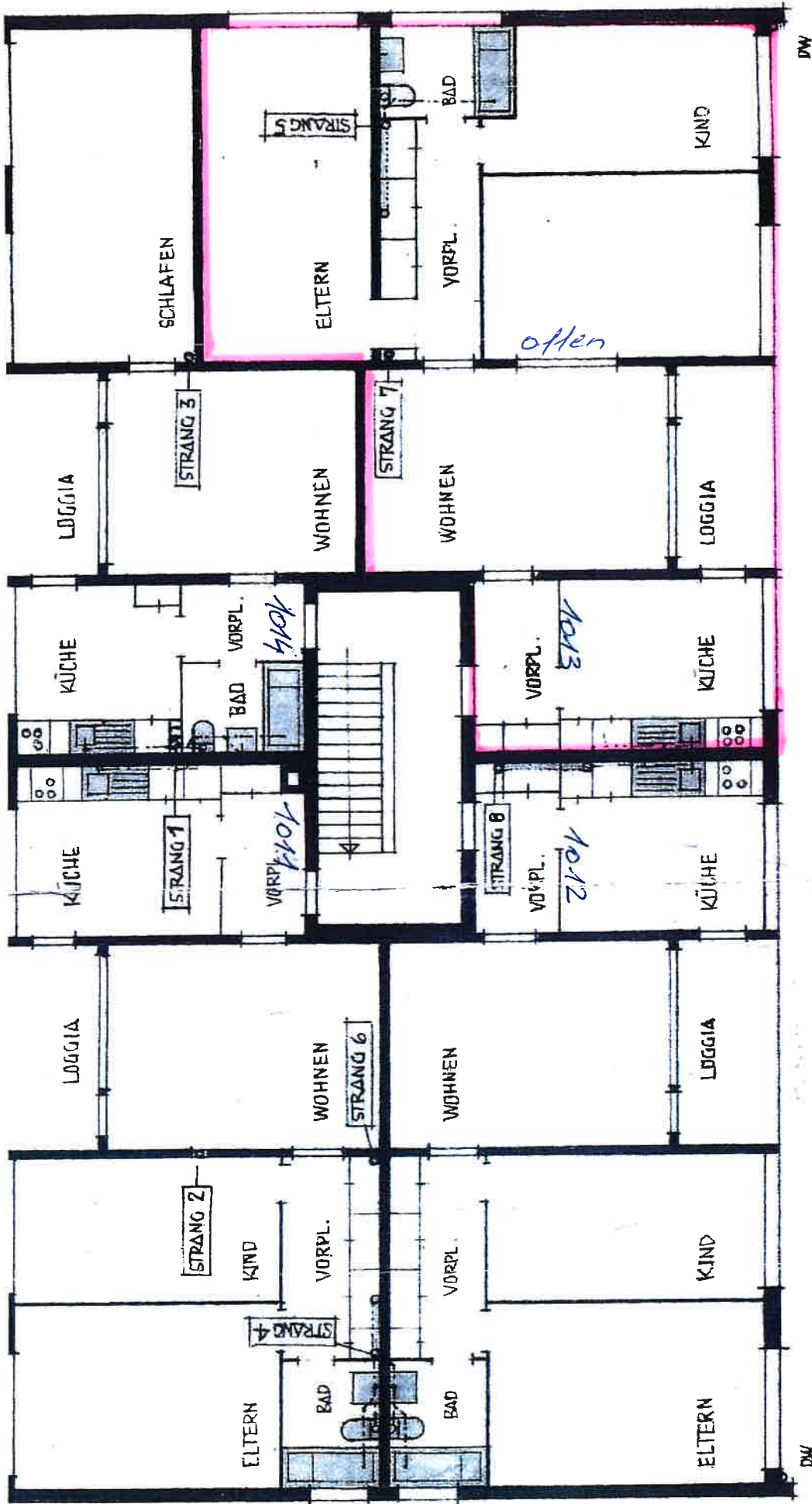
OBERGESCHOSS 1:100
