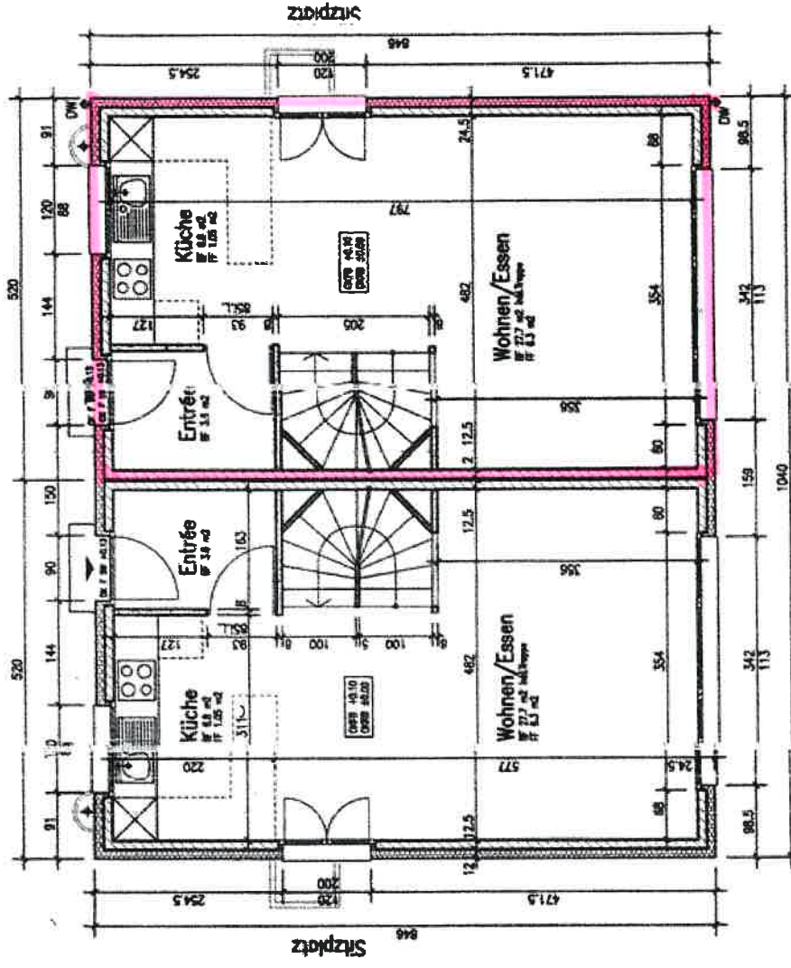
Haus Erdgeschoss
