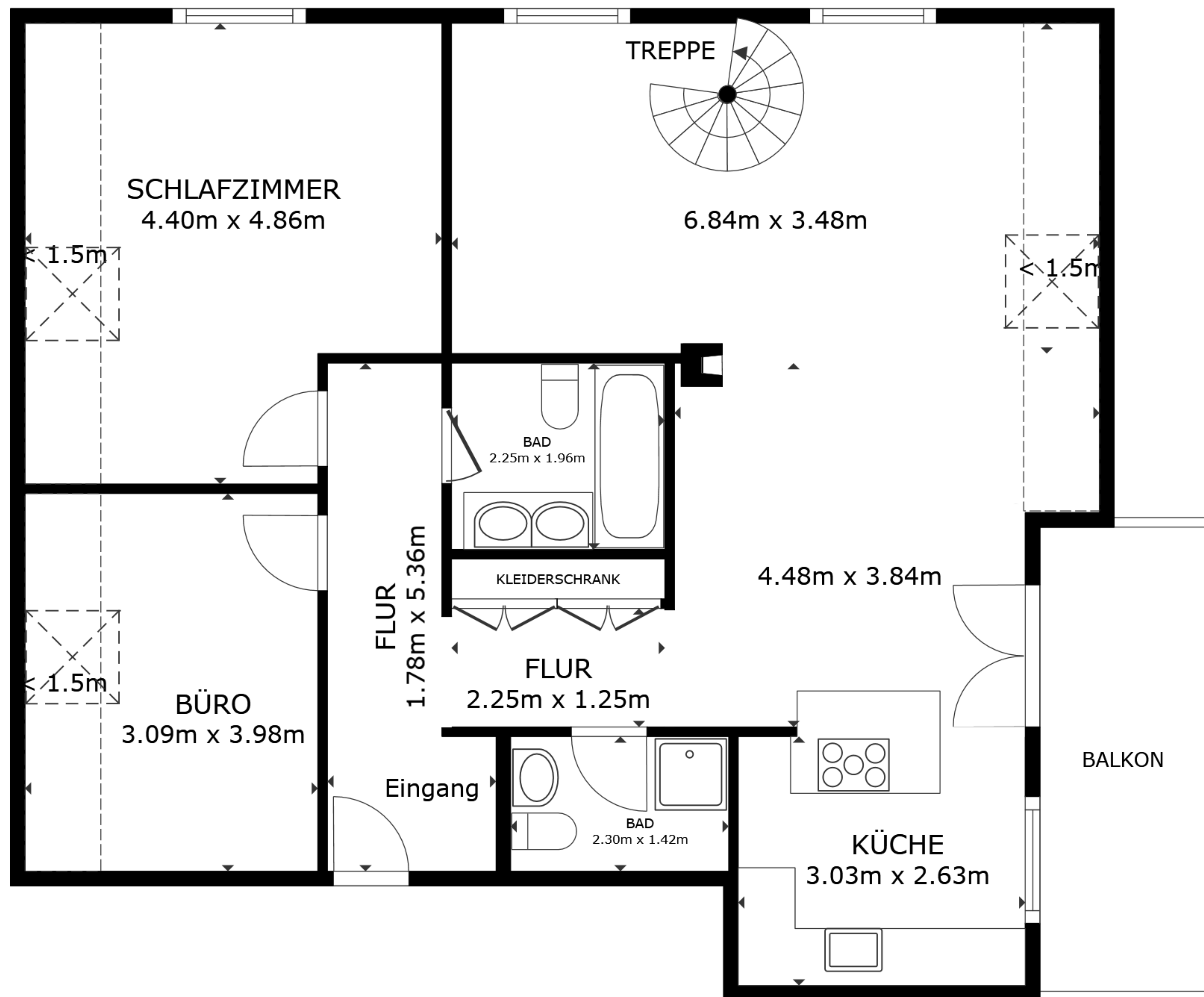
STOCKWERK 1
