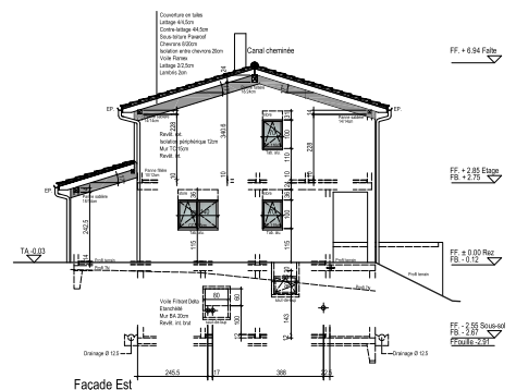
Façade Est
