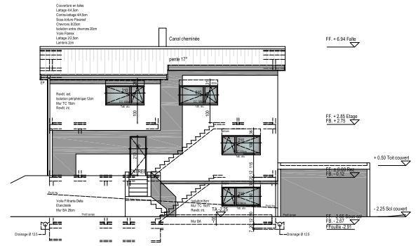
Façade Nord
