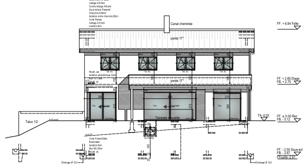
Façade Sud
