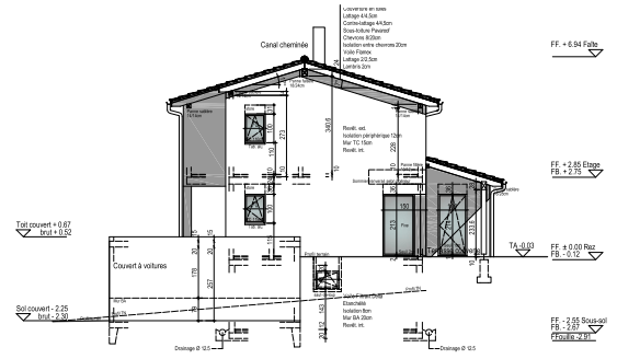
Façade Ouest
