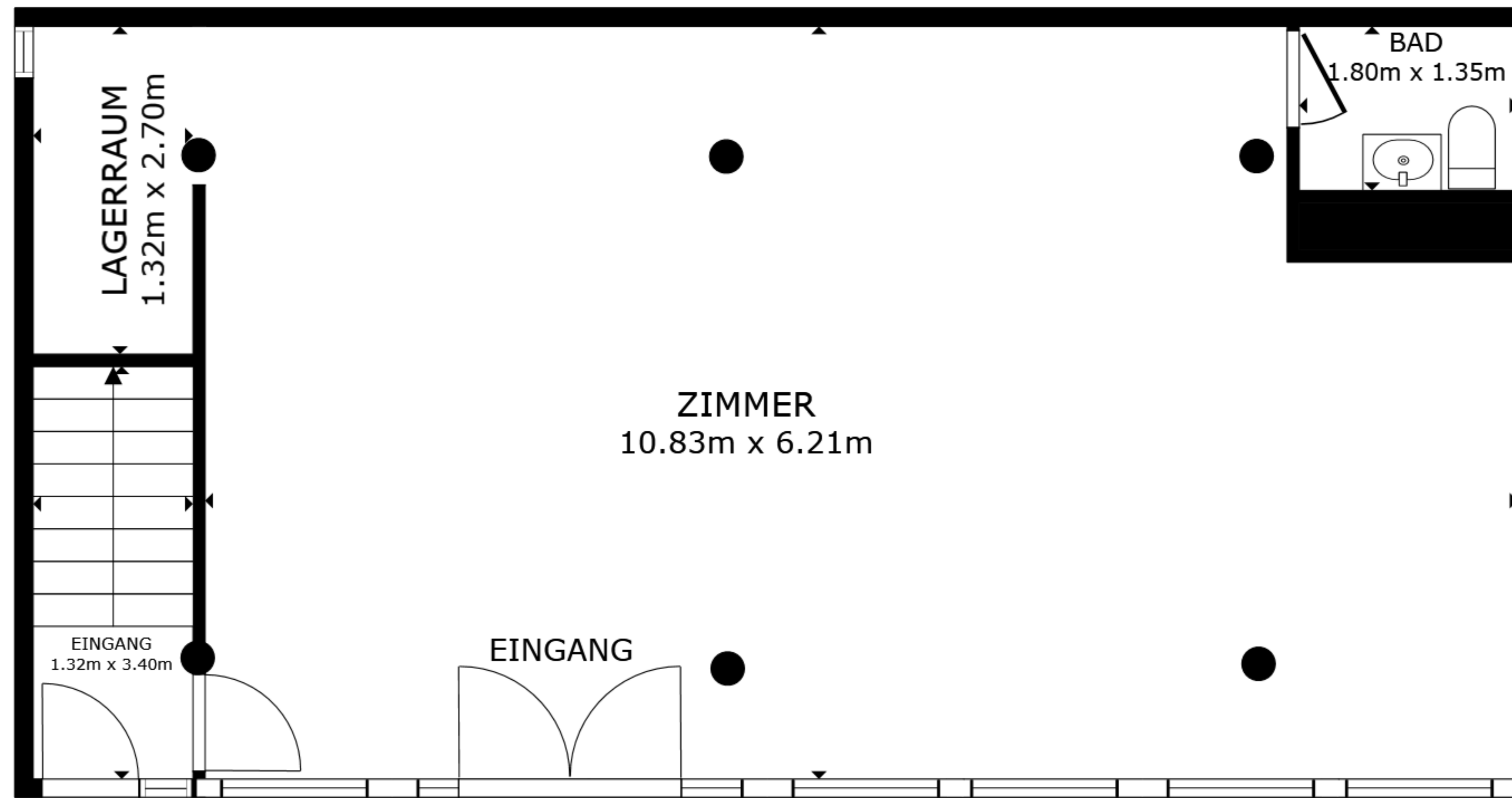
STOCKWERK 1
