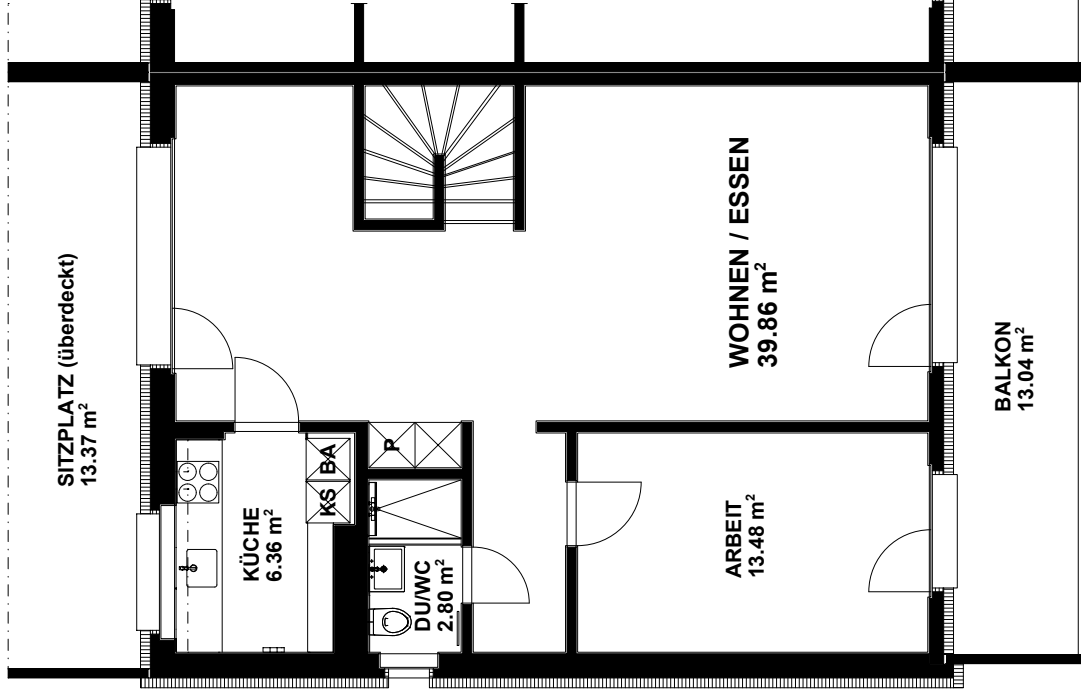
Obergeschoss 1:100
