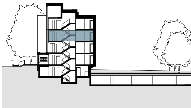
SCHEMASCHNITT
