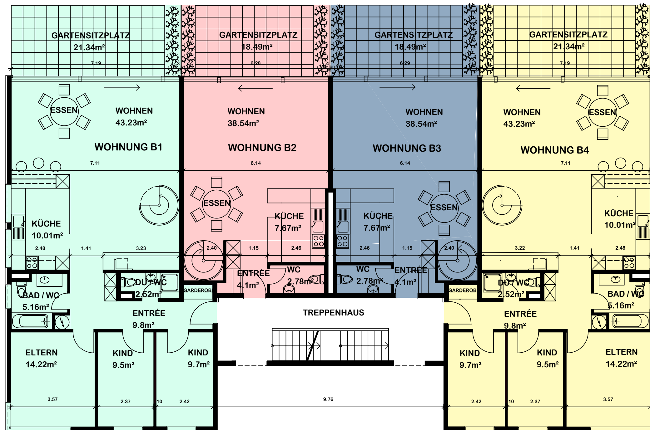
TERRASSENWOHNUNGEN IN IPSACH BUCHENWEG 7. ERDGESCHOSS M. 1:100 HOHL+ PARTNER IPSACH 032 331 70 88
