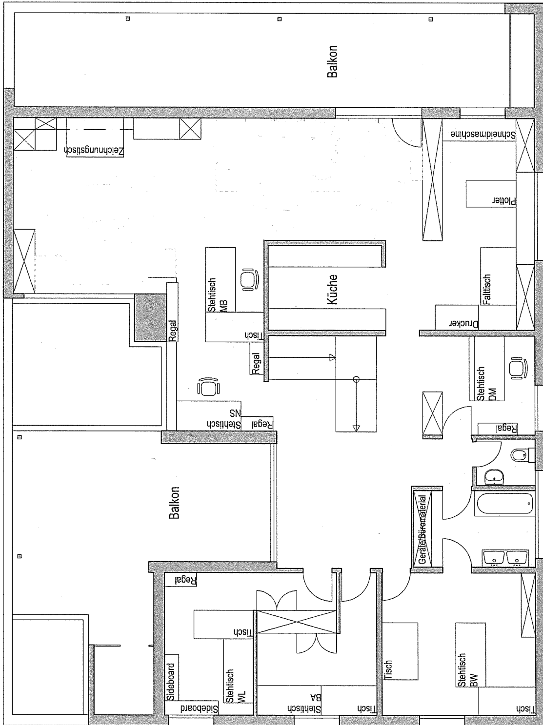
Obergeschoss
