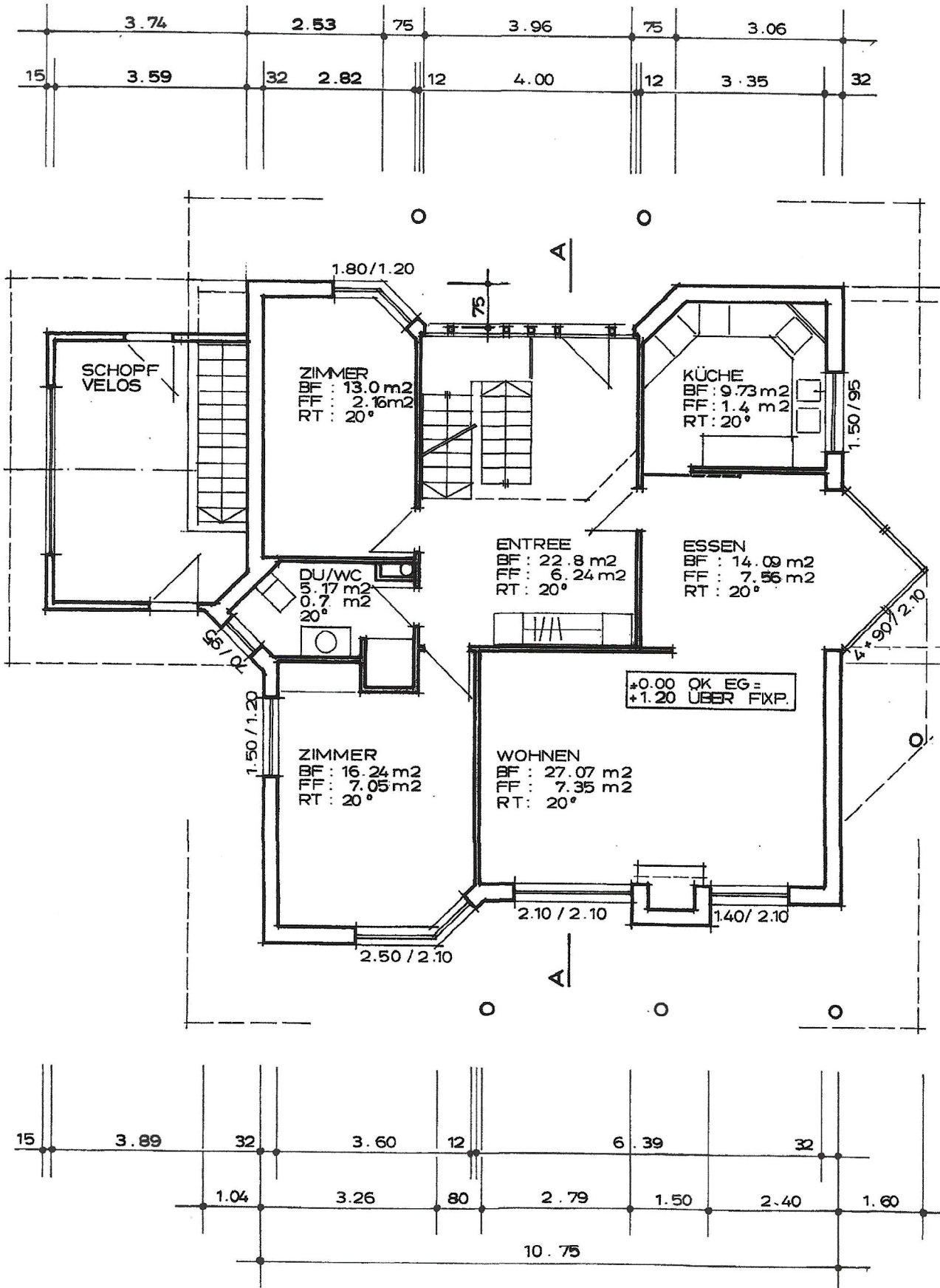
GRUNDRISS ERDGESCHOSS
