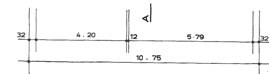
GRUNDRISS OBERGESCHOSS
