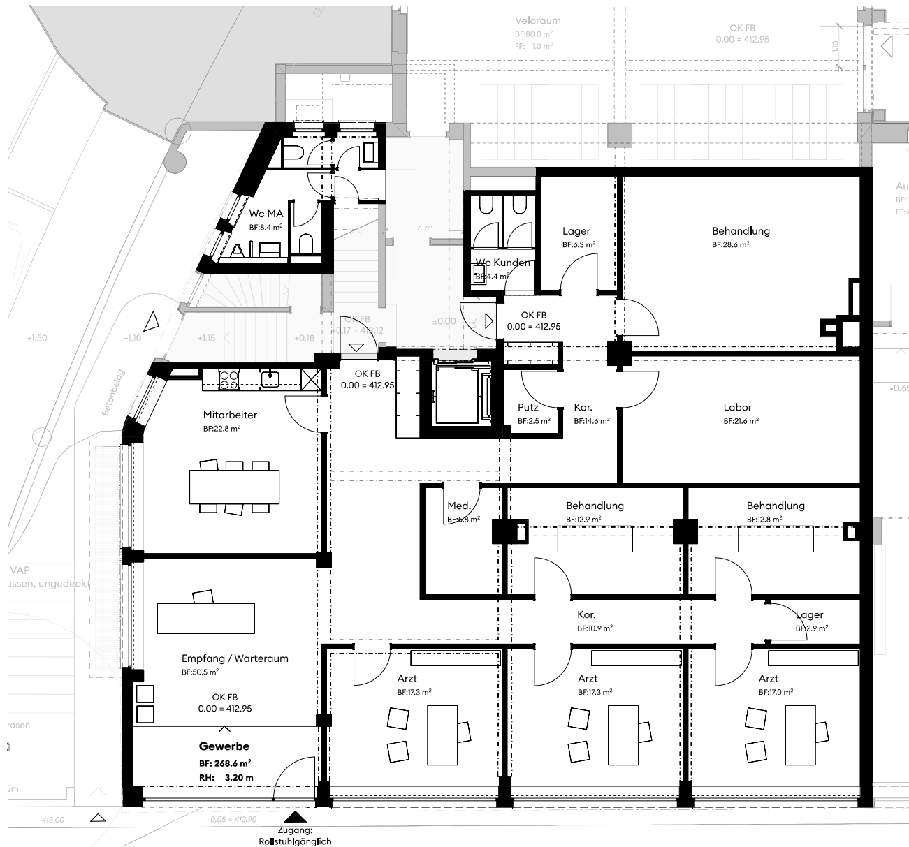
Grundriss 1:100
