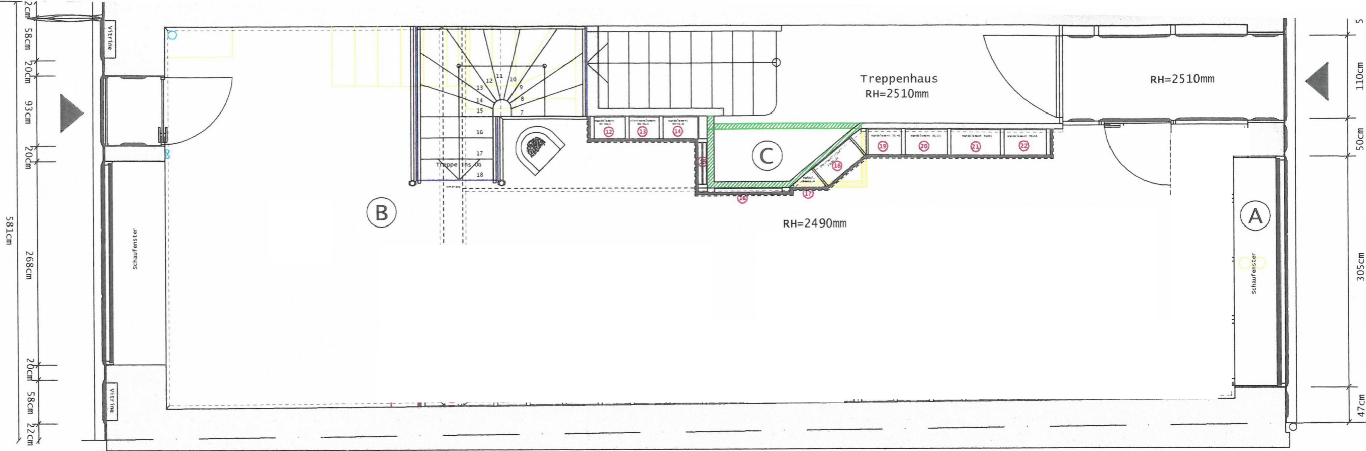
Grundriss Erdgeschoss/L-A/1:50
