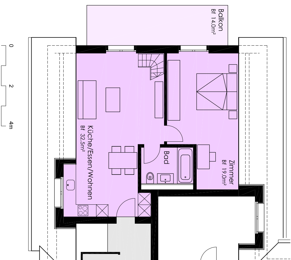
1. Dachgeschoss
