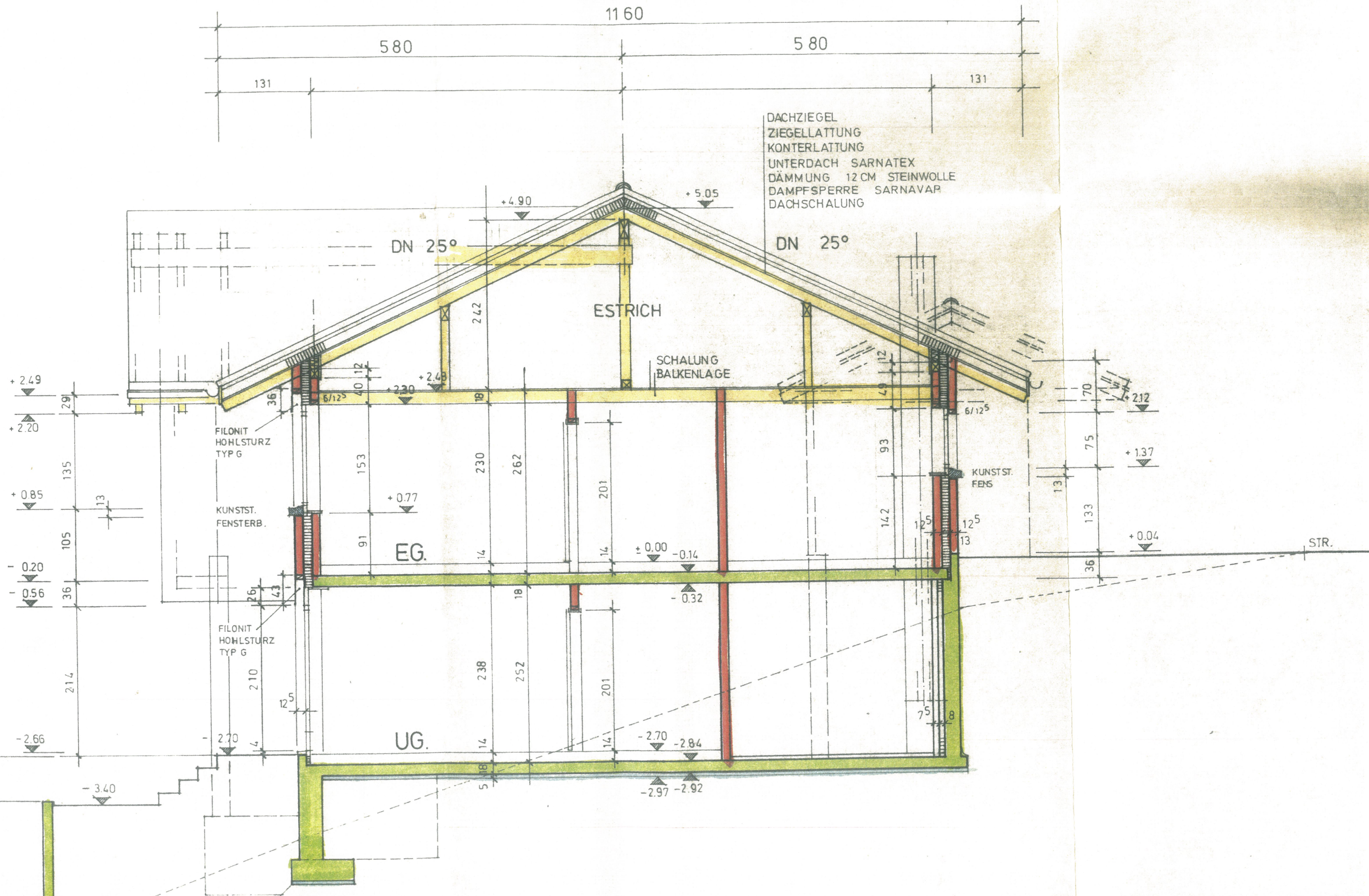
QUERSCHNITT A-A
