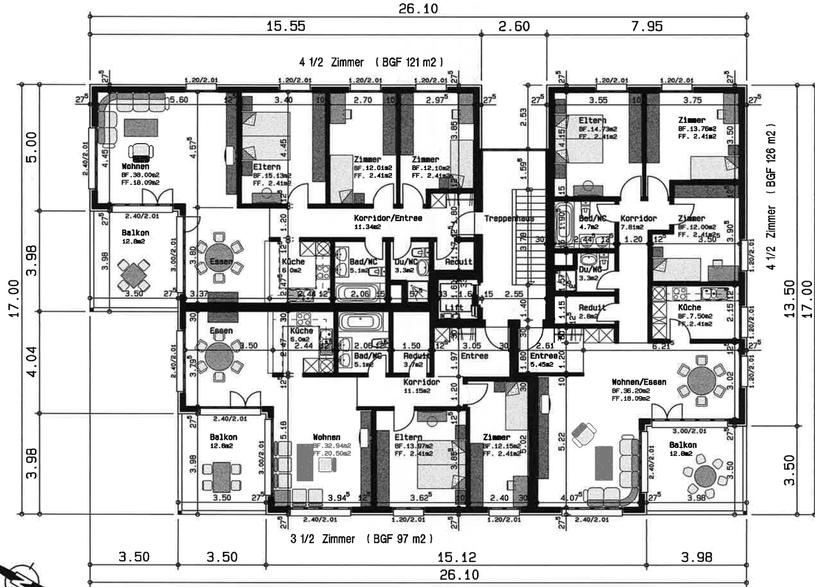
Grundriss 1.-3.Obergeschoss
