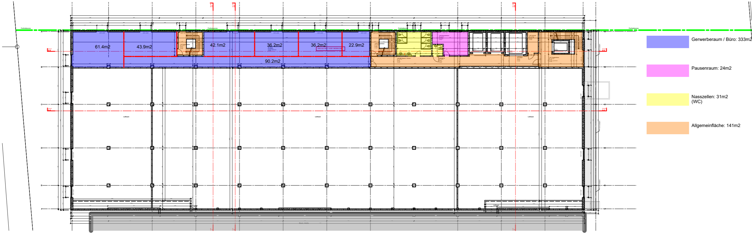
Erdgeschoss Ebene 2
