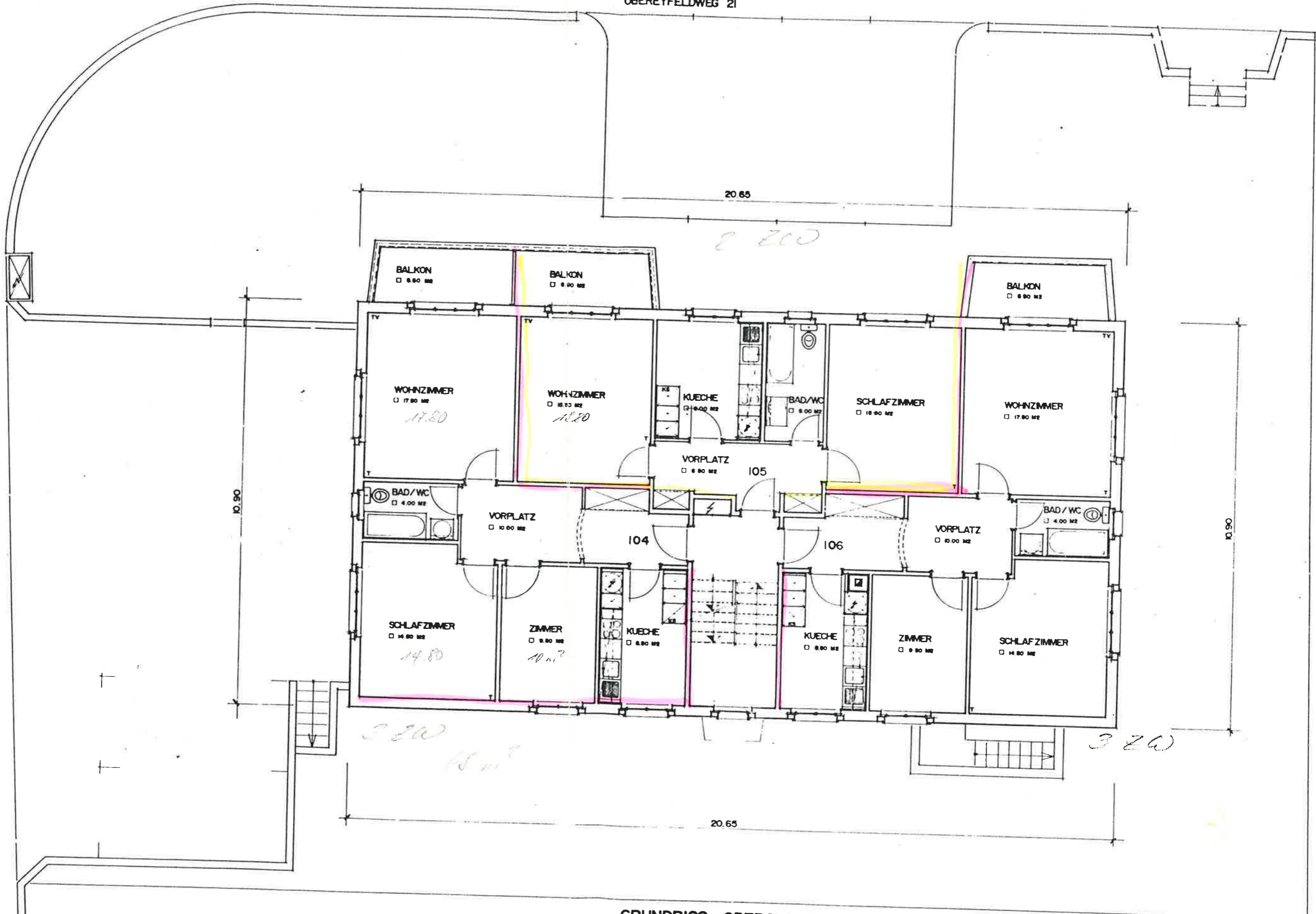
GRUNDRISS OBERGESCHOSS
