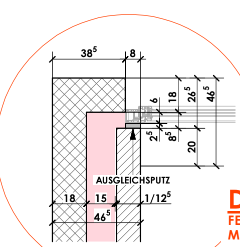
DETAIL A Fenster-/Türanschlag MST. 1:20
