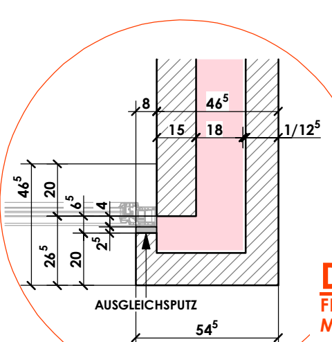
DETAIL B Fenster-/Türanschlag MST. 1:20
