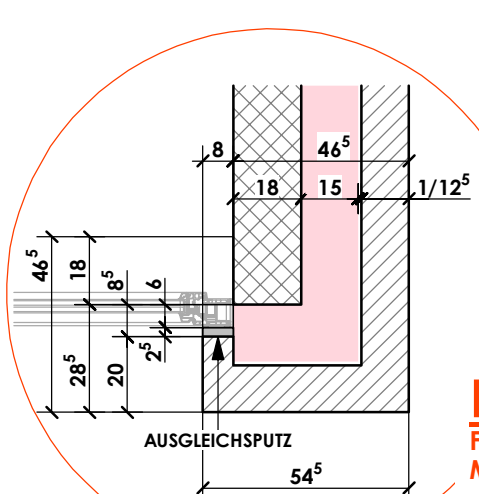
DETAIL C Fenster-/Türanschlag MST. 1:20
