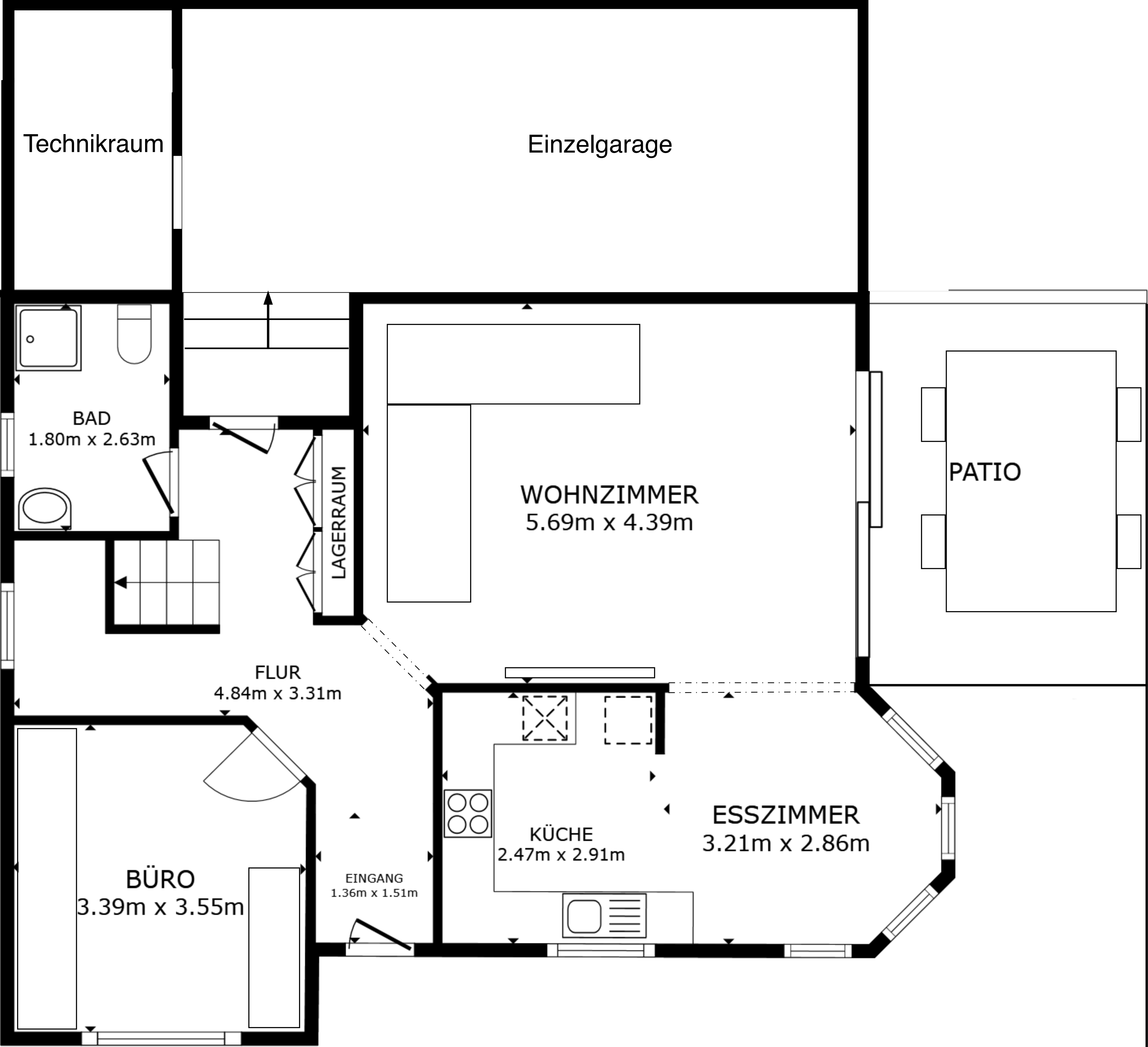
STOCKWERK 1
