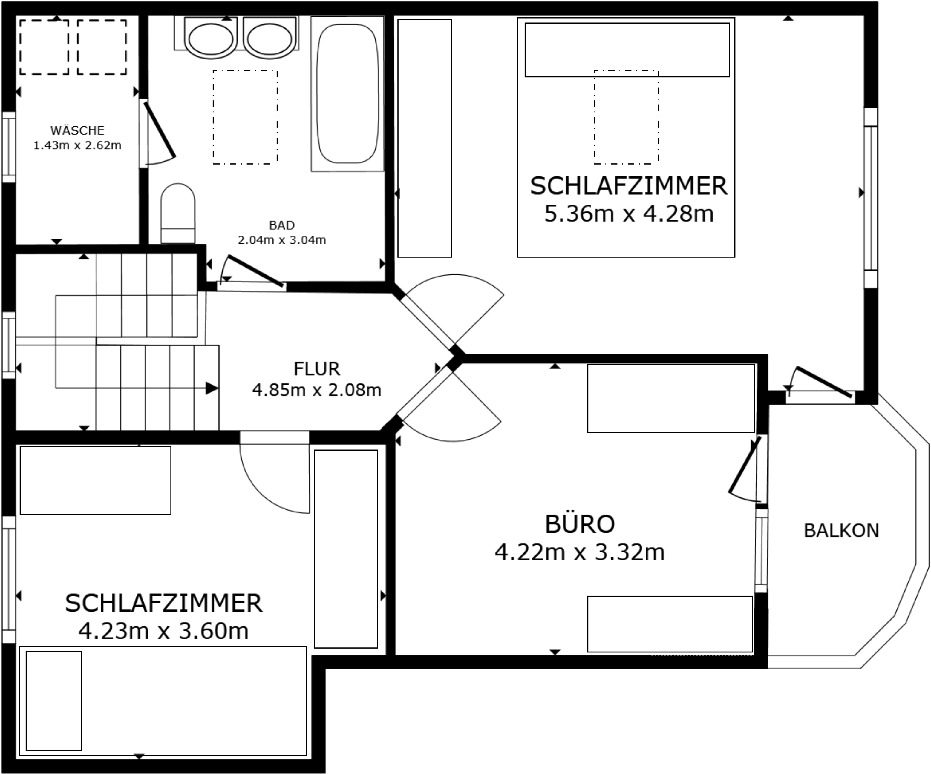
STOCKWERK 2
