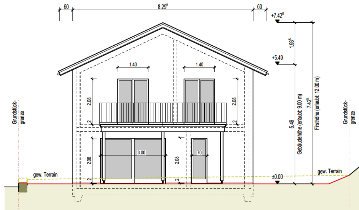
Südfassade
