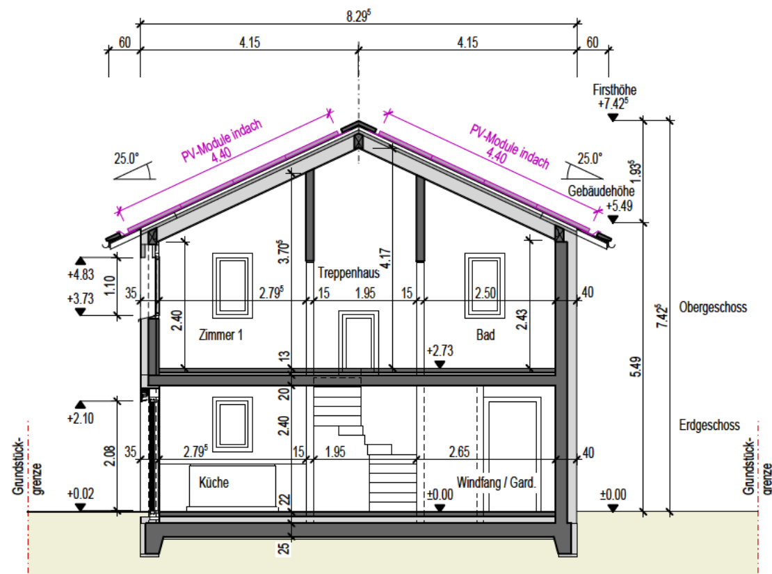
Schnitt
