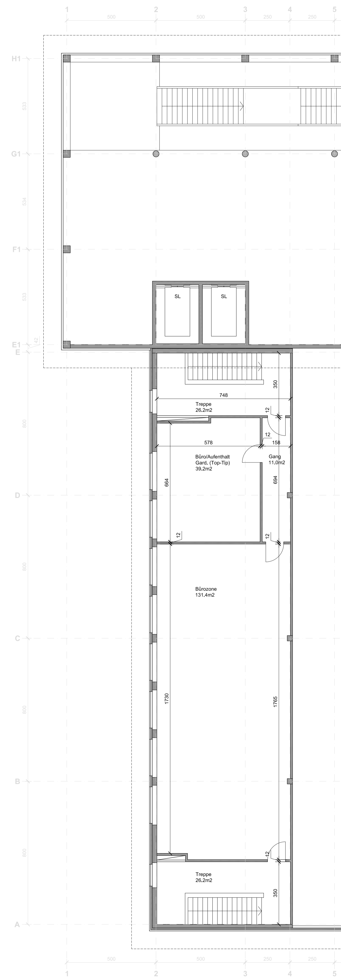
OG Zwischengeschoss
