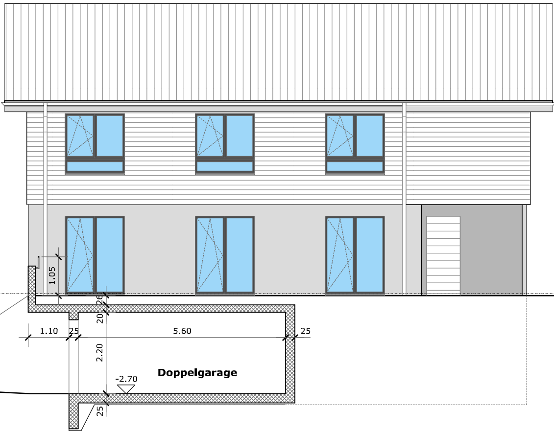
Fassade Ost
