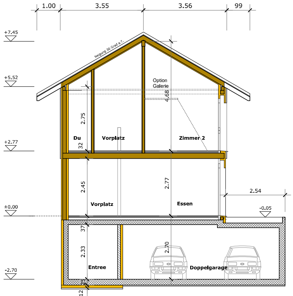
Querschnitt
