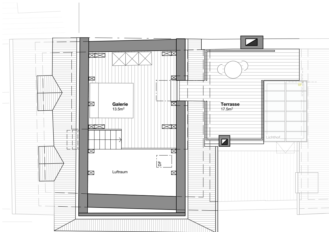
Galerie
