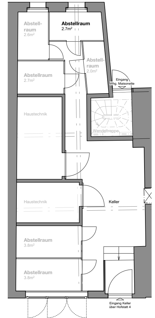
Untergeschoss
