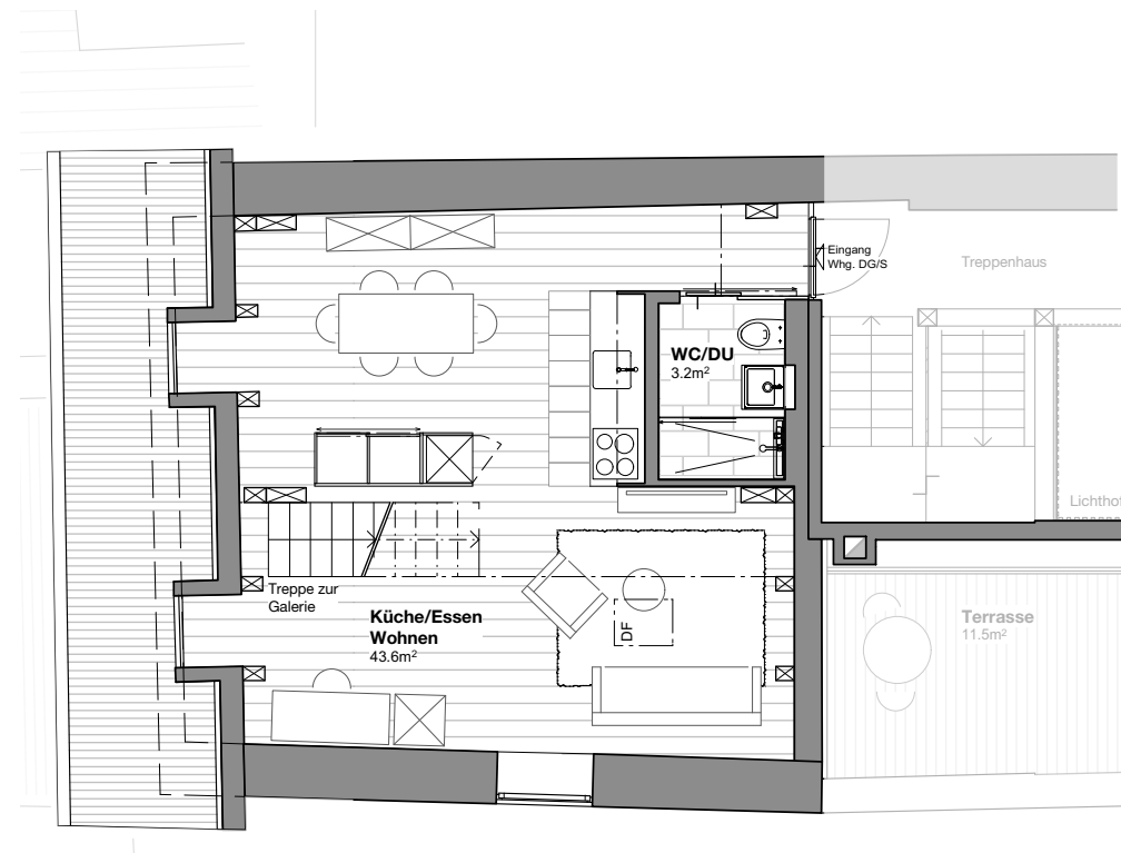
Dachgeschoss
