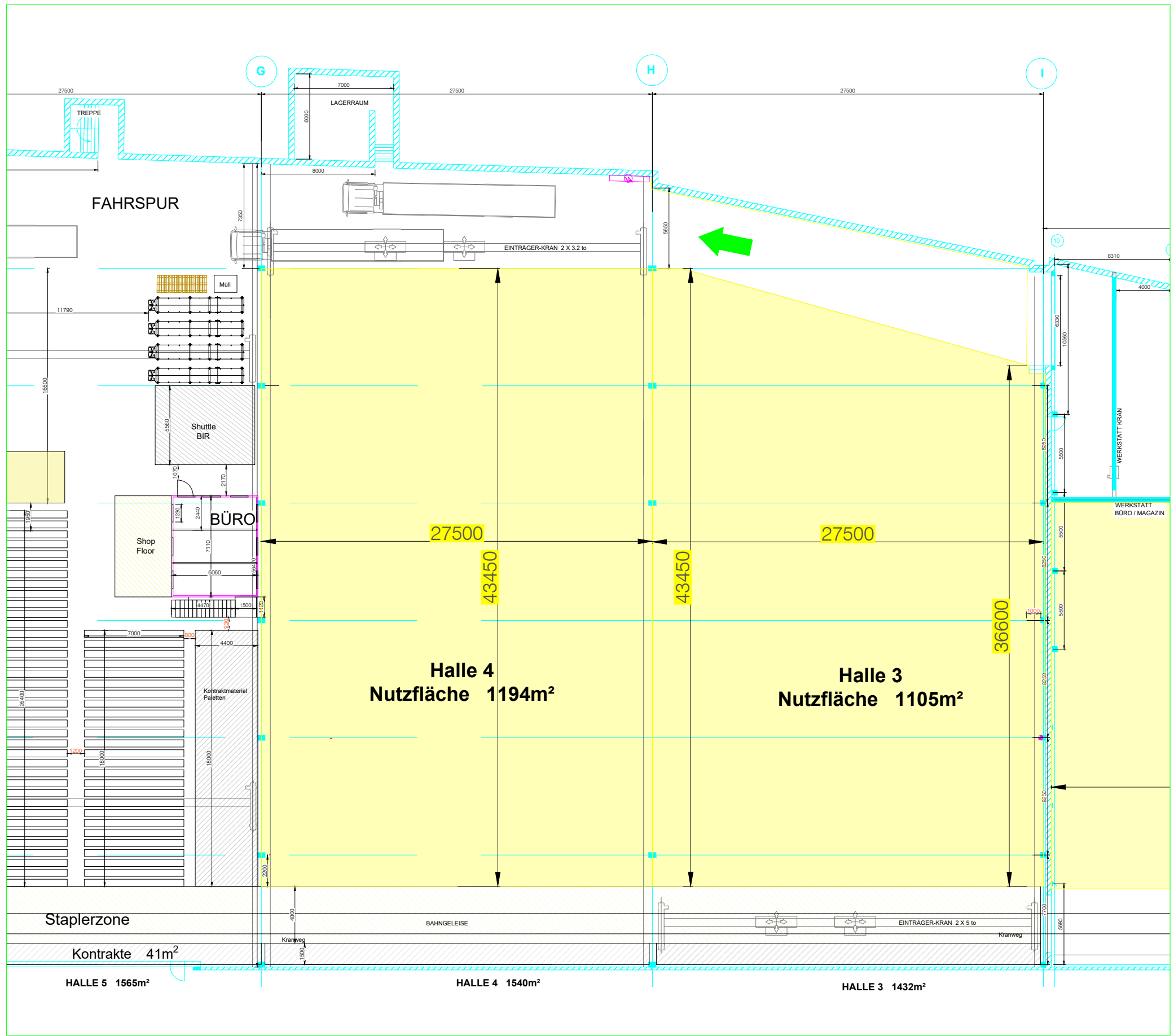
Debrunner St.Gallen Halle 3-4 A3 / M1:300 11.01.2024
