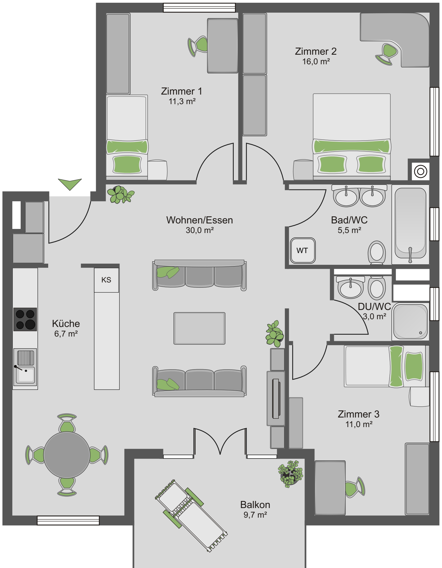
1. Obergeschoss Nr. 111
