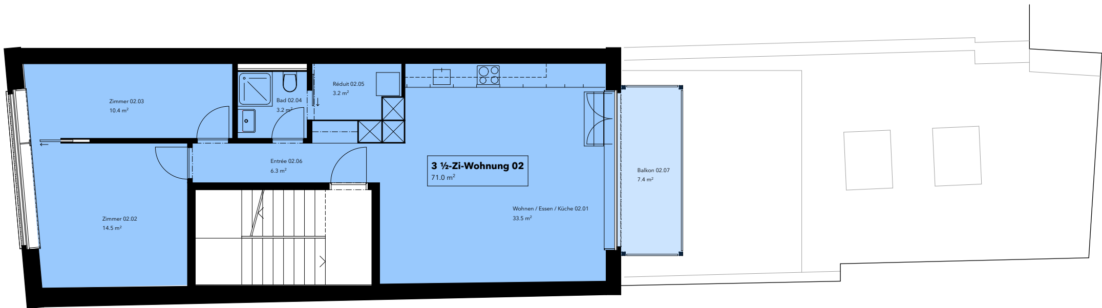
2. Obergeschoss: Wohnung 02
