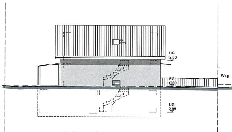
Russikerstrasse 17 Ostfassade
