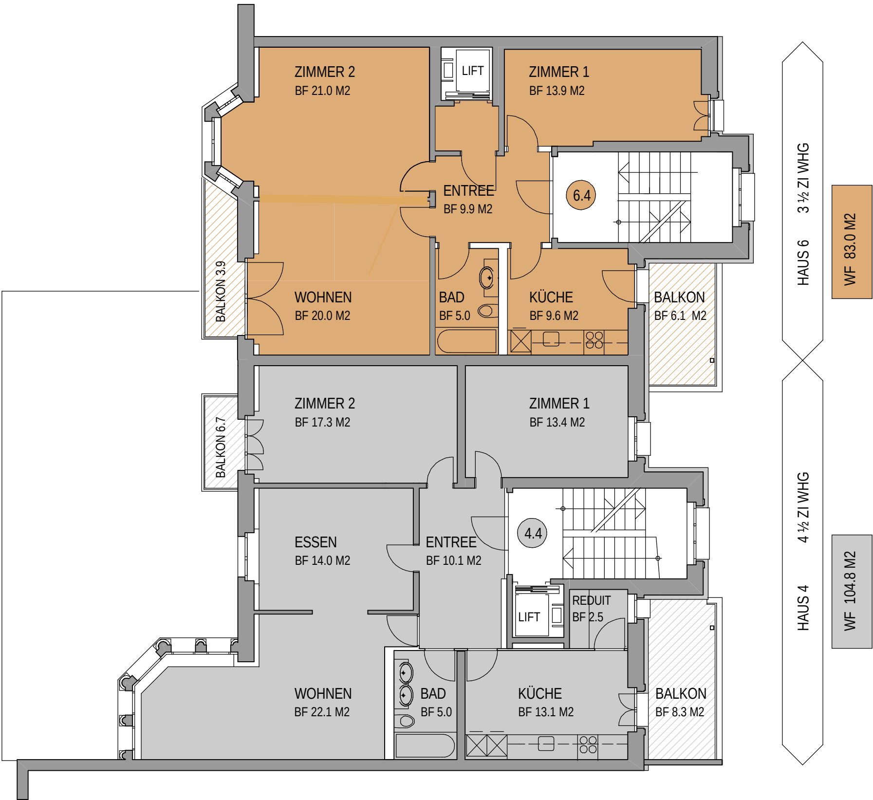
GRUNDRISS 4. OBERGESCHOSS 1 : 100
