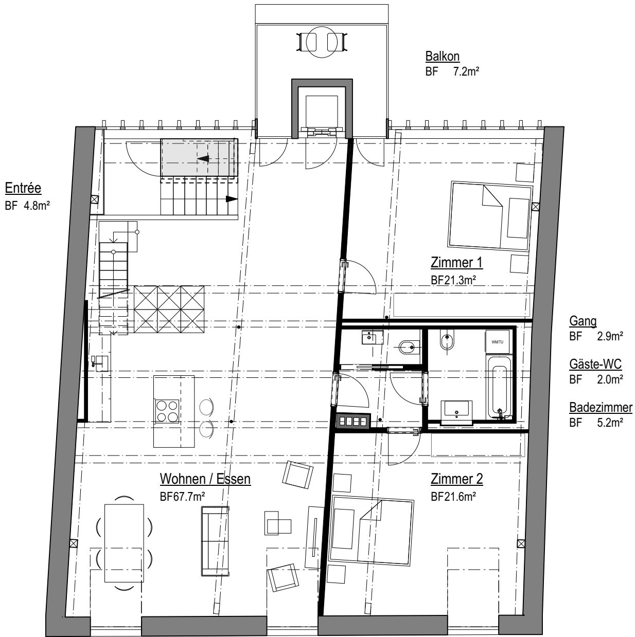
Dachgeschoss
