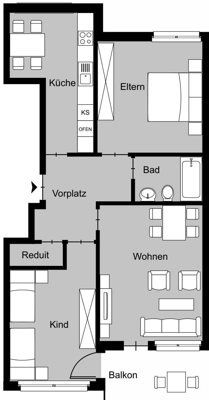
Obergeschoss
