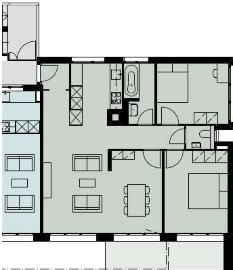
Whg. 3.6. 3.5-Zimmer-Wohnung NWF: 81.33 m 2
