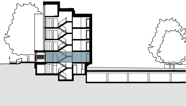
SCHEMASCHNITT
