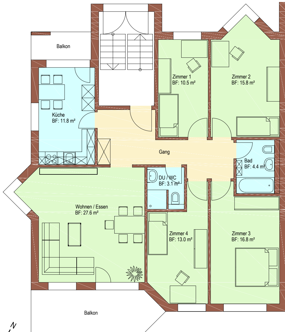
Wohnungstyp W15 5.5 Zimmer Wohnung ca. 115 m² Nr. 12, 26
