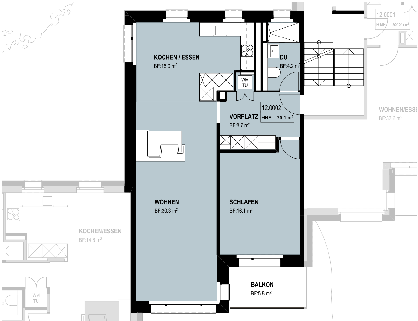
GRUNDRISS
