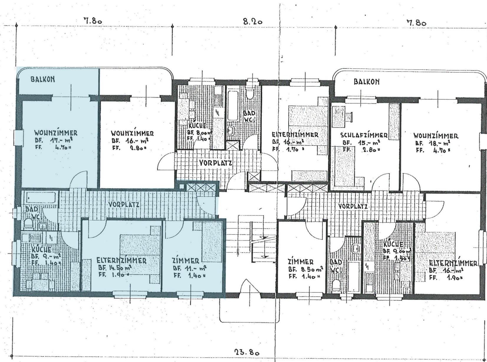
GRUNDRİSS : PARTERRE, 1. u. 2. STOCK
