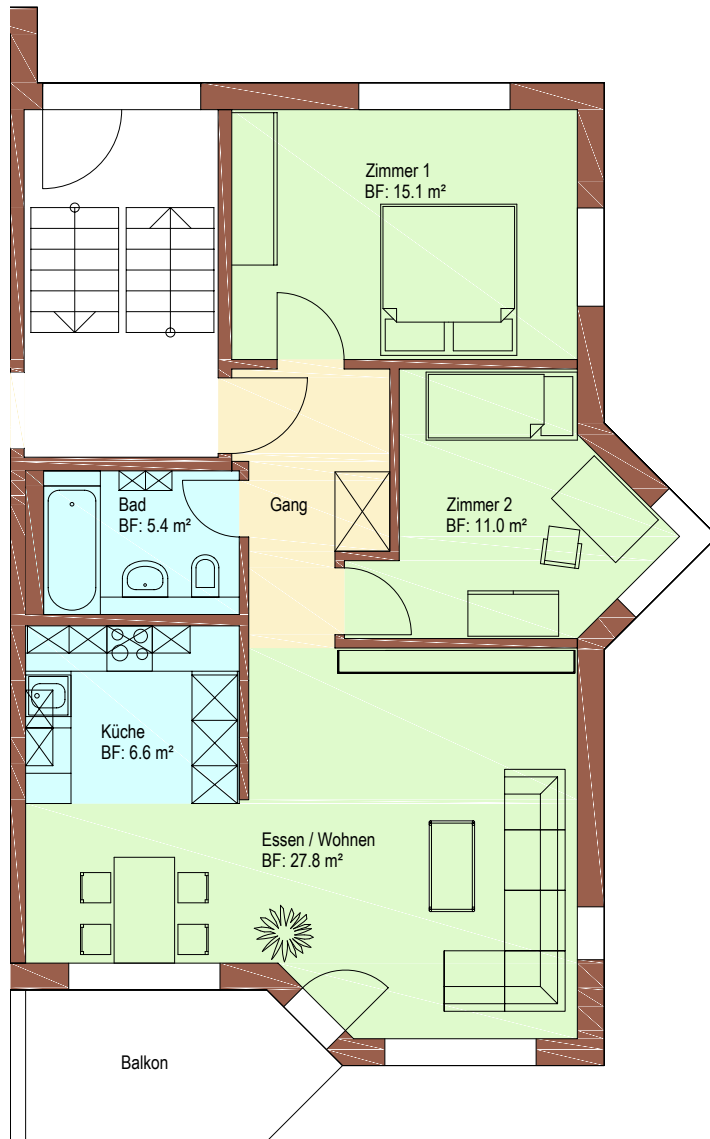
Wohnungstyp W10 3.5 Zimmer Wohnung ca. 71 m 2 Nr. 2, 5, 16, 19
