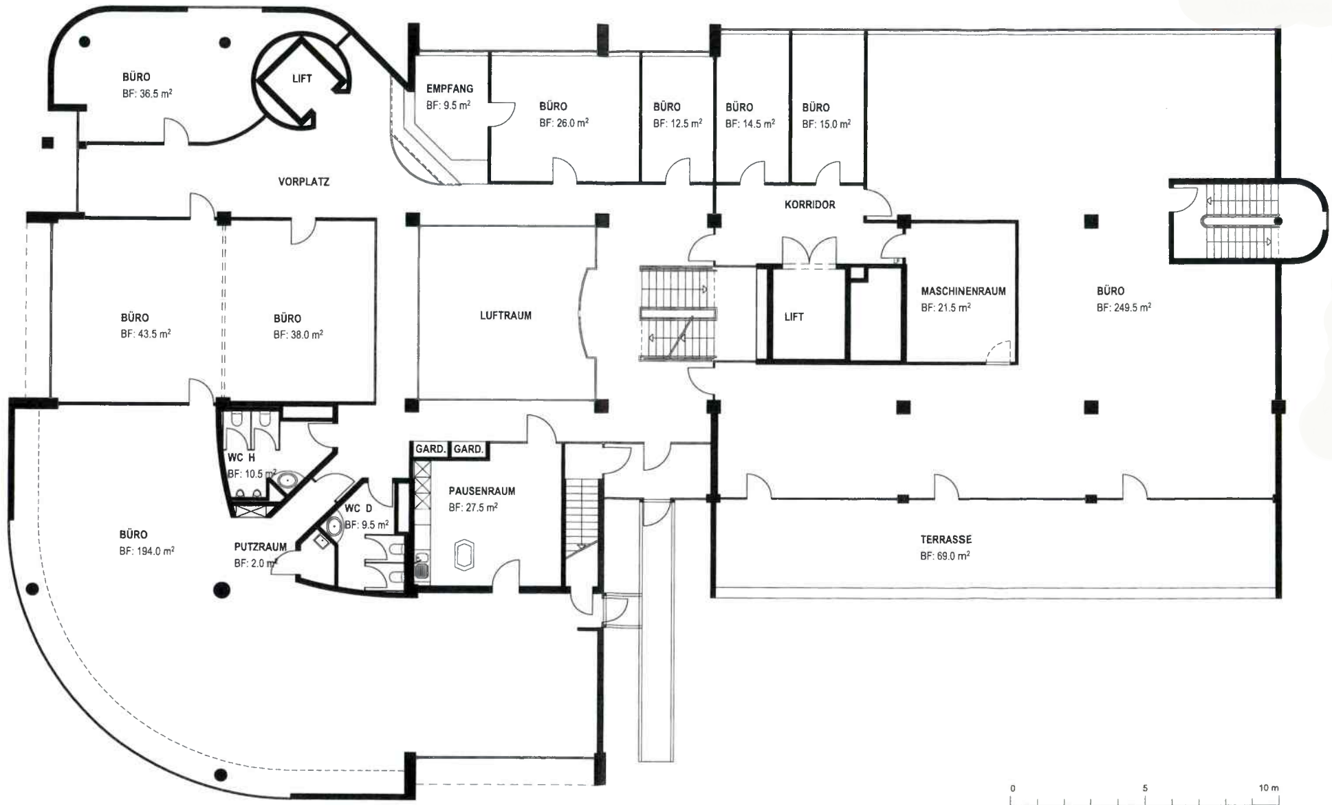
1. OBERGESCHOSS
