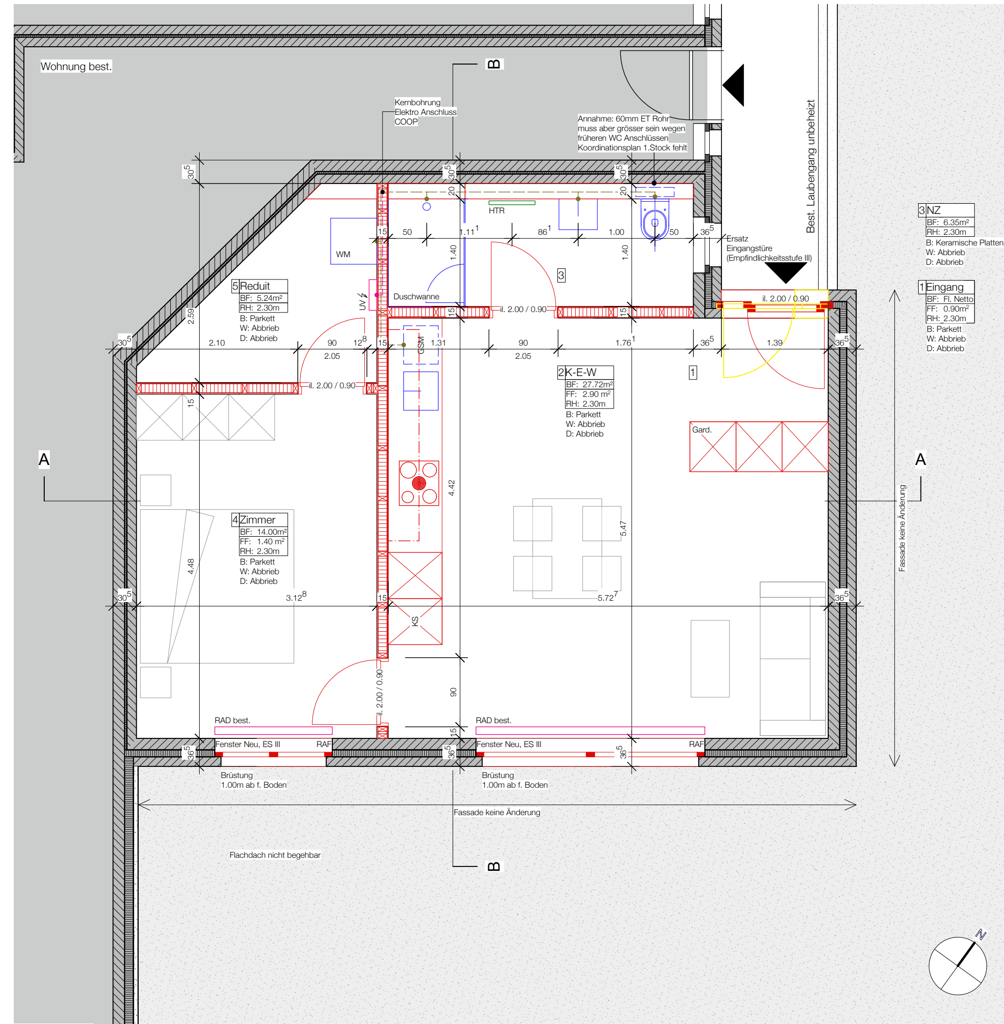
Grundriss
