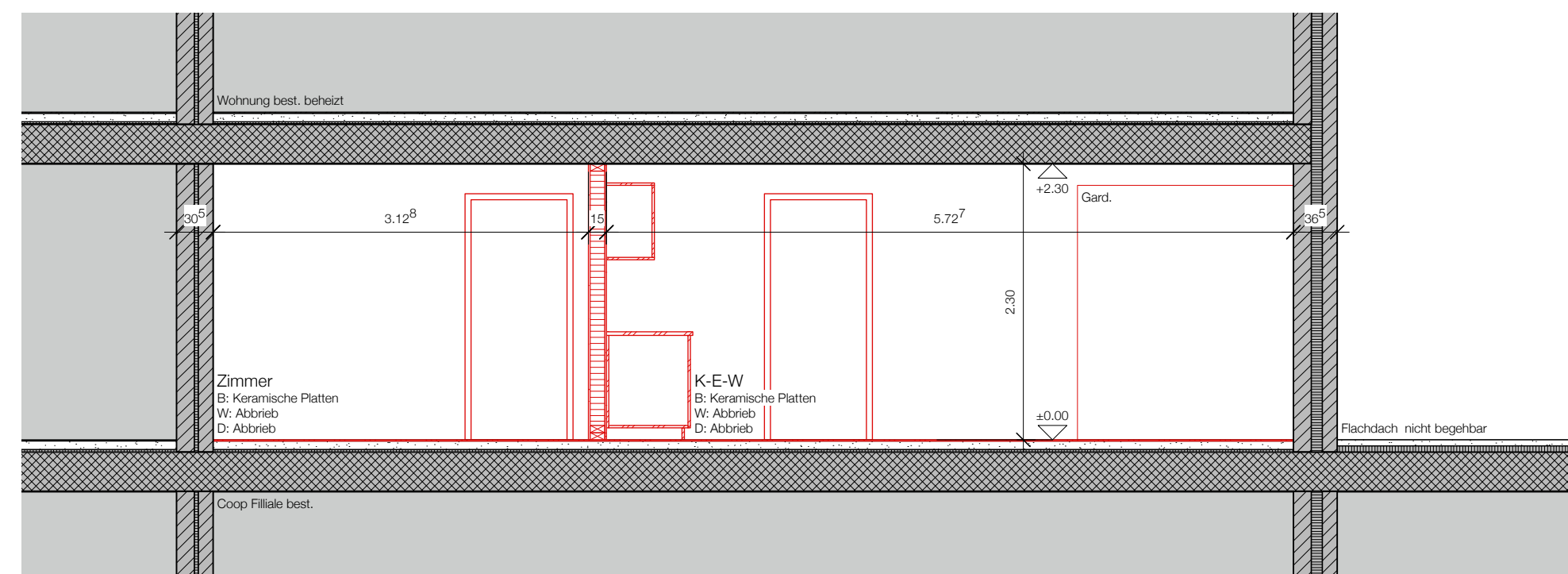
Schnitt A
