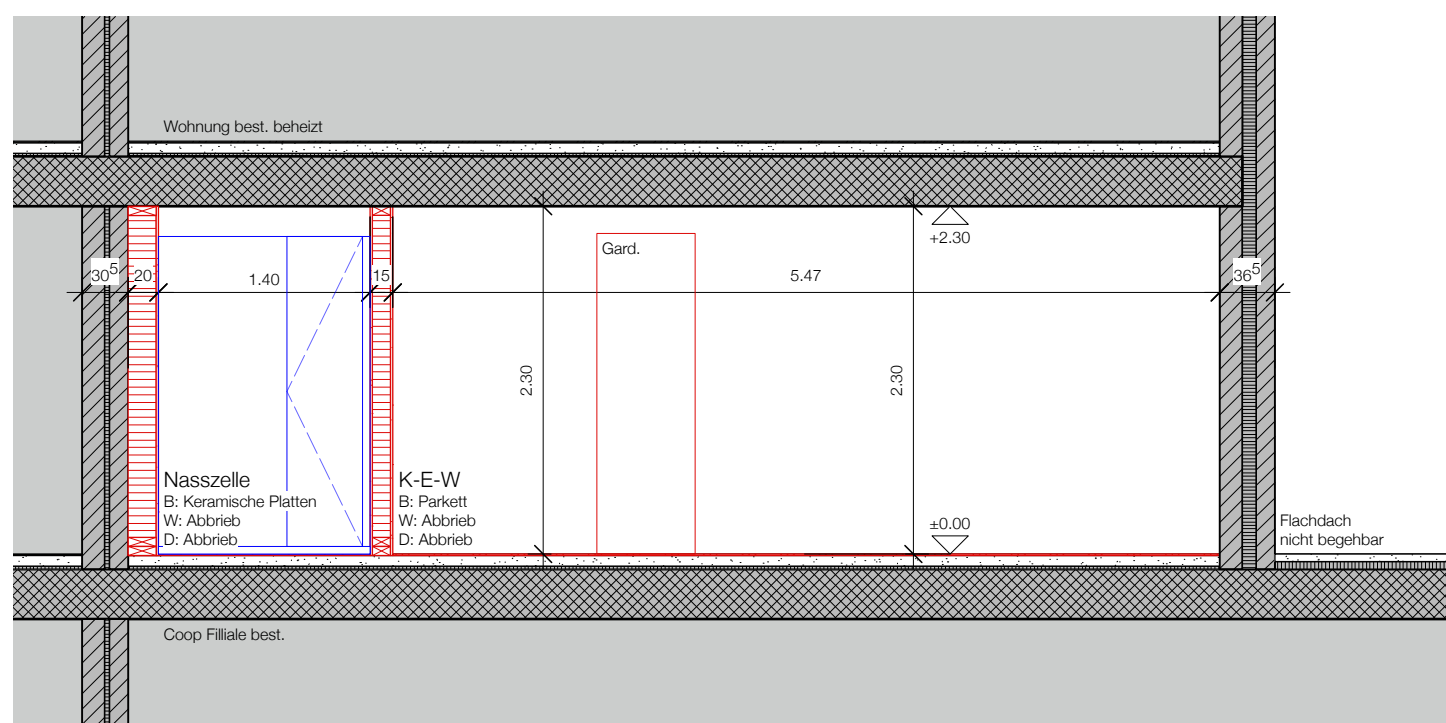
Schnitt B
