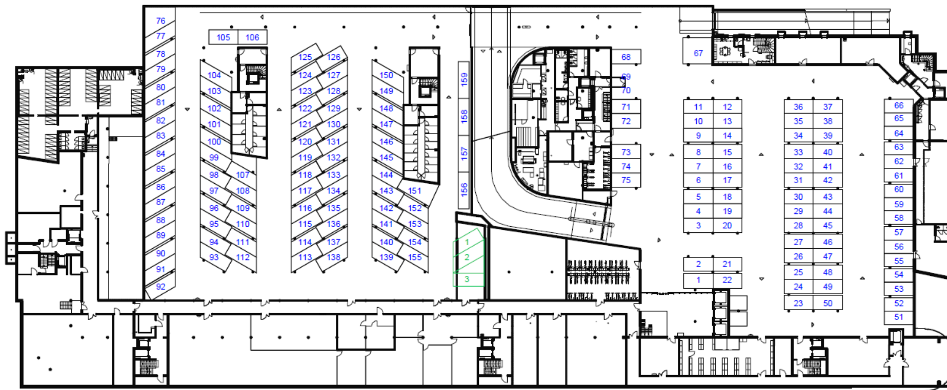
Parkgeschoss 1, 1:700
