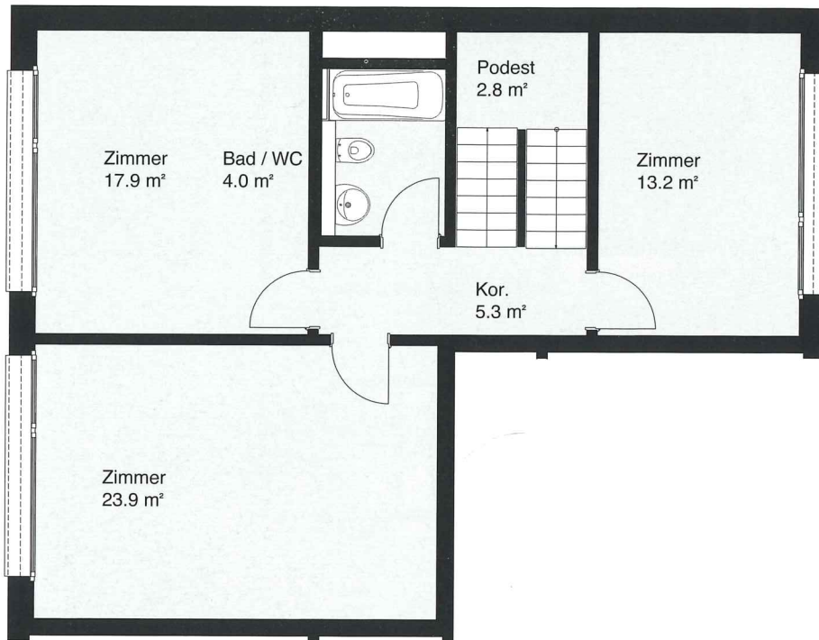
1. Obergeschoss
