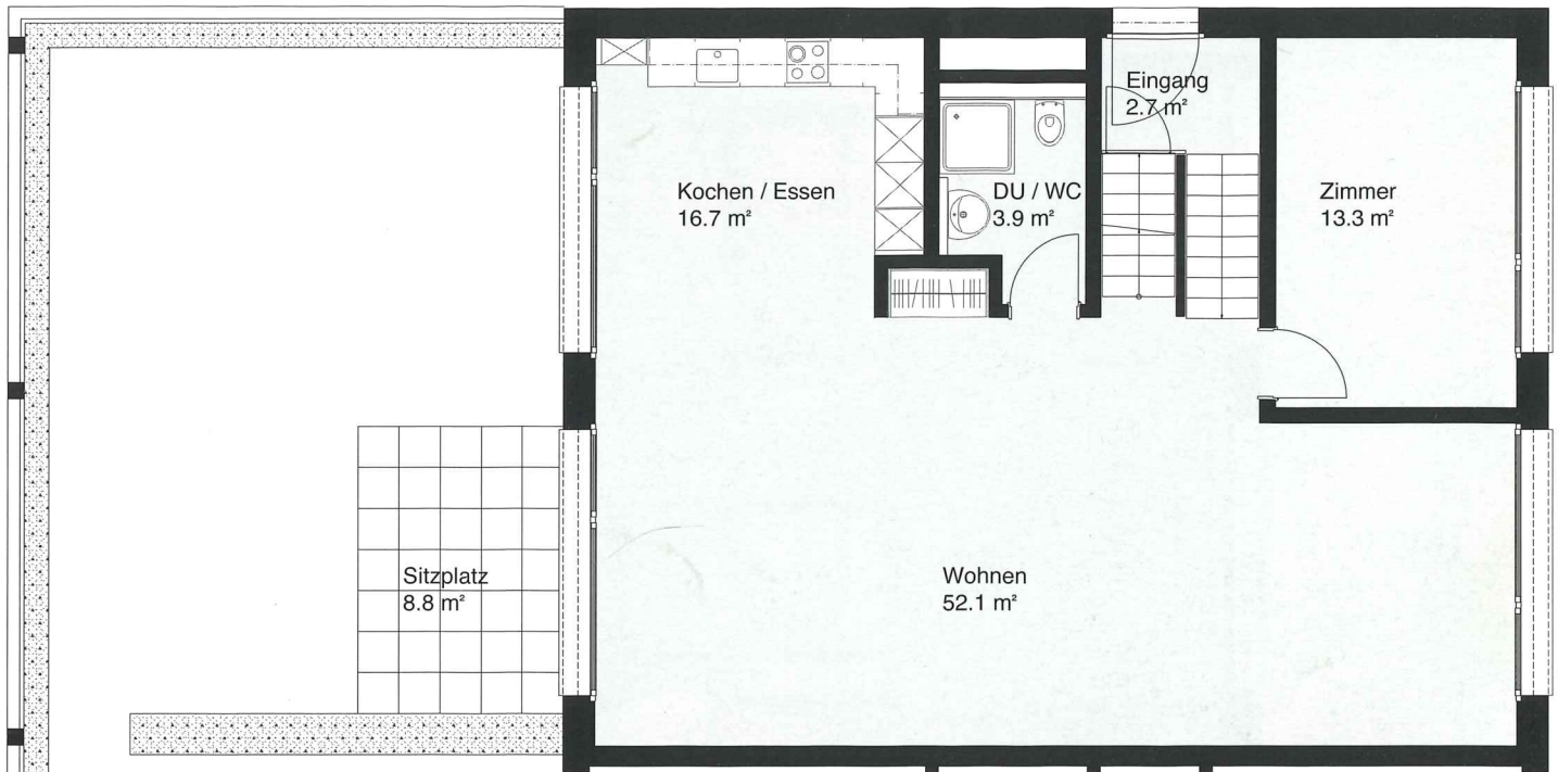
Erdgeschoss
