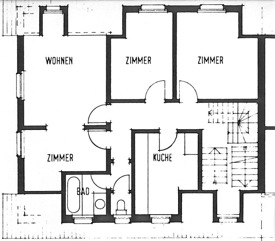
DACHGESCHOSS 1
