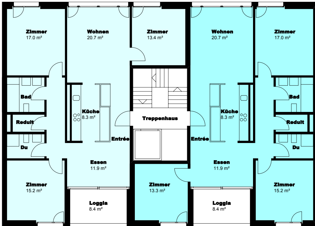
Grundriss M. 1:150
